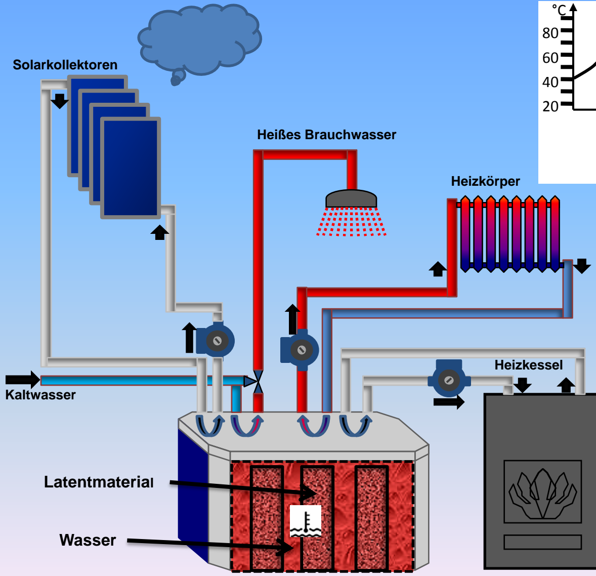
POMOSYS ® HYBRIDWÄRMESPEICHER
