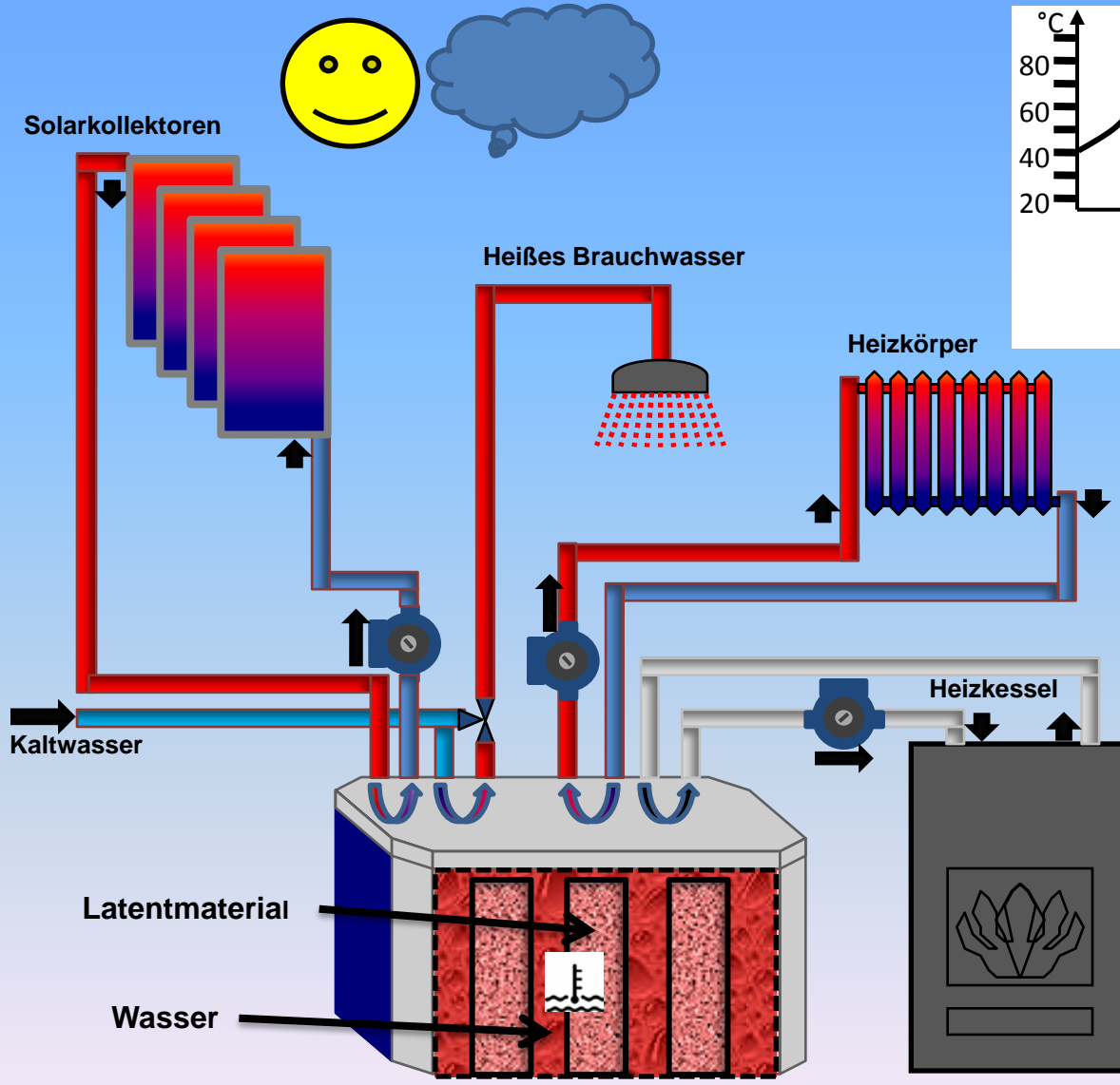
POMOSYS ® HYBRIDWÄRMESPEICHER
